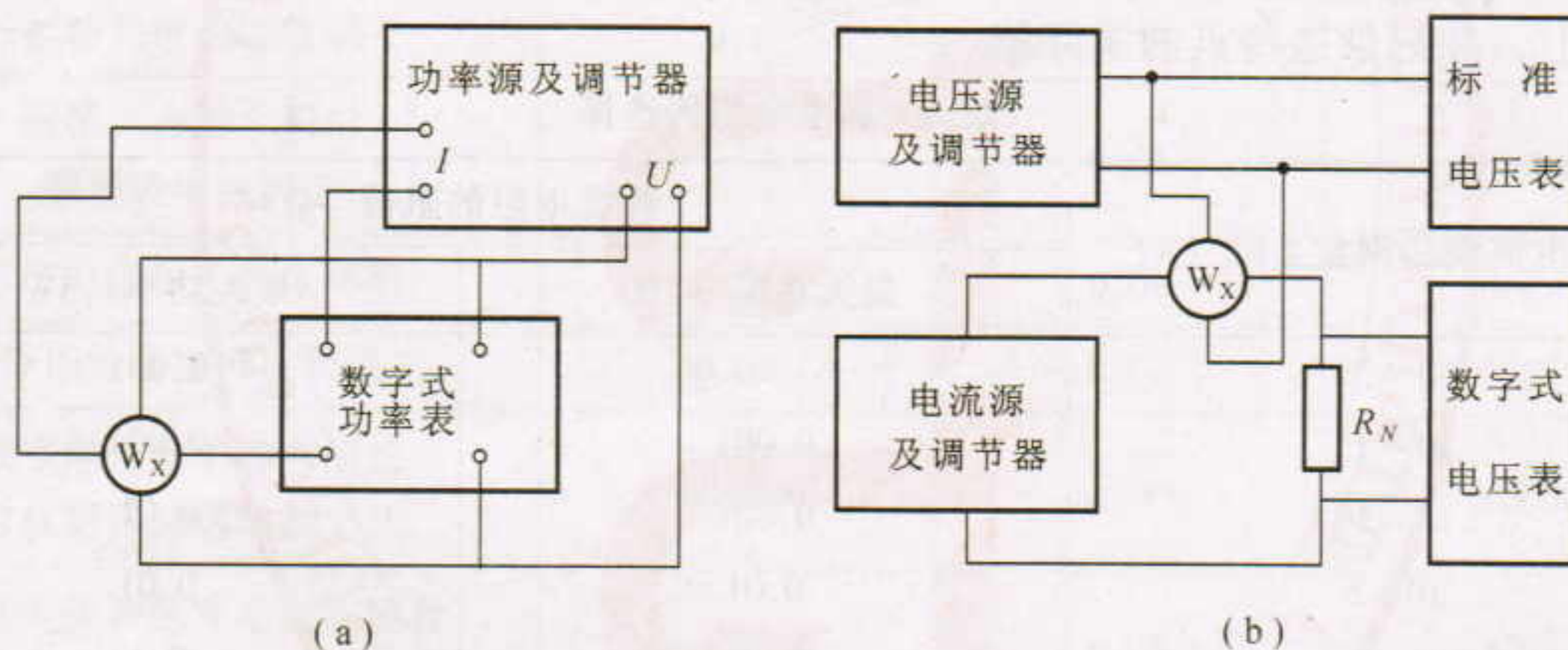
图3 用数字表检定功率表的接线图
