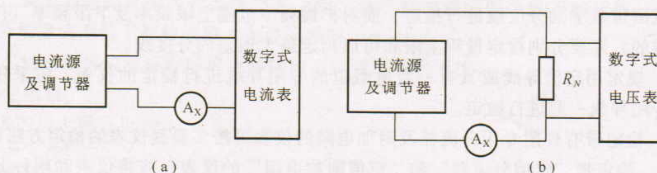
图 1 用数字表检定电流表的接线图
