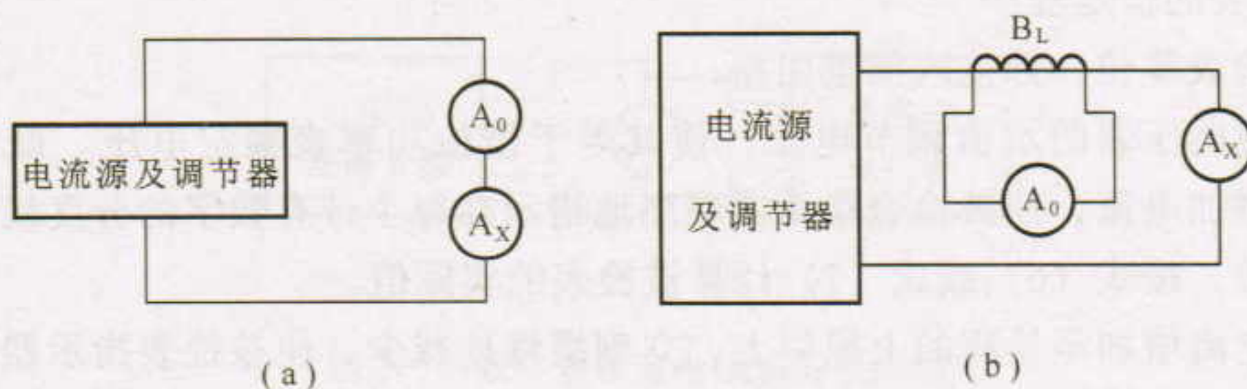
图4 检定电流表的接线图
