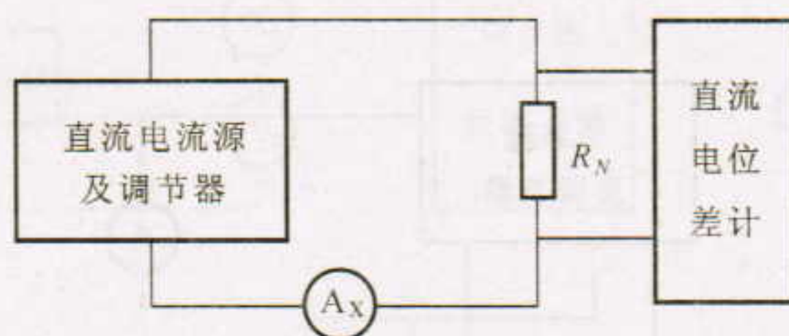
图 7 检定直流电流表的接线图
