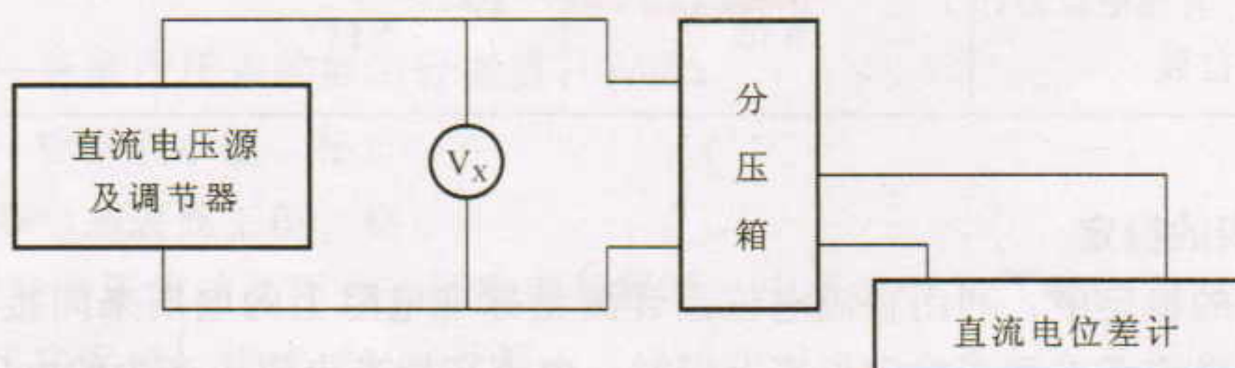
图 9 检定直流电压表的接线图
