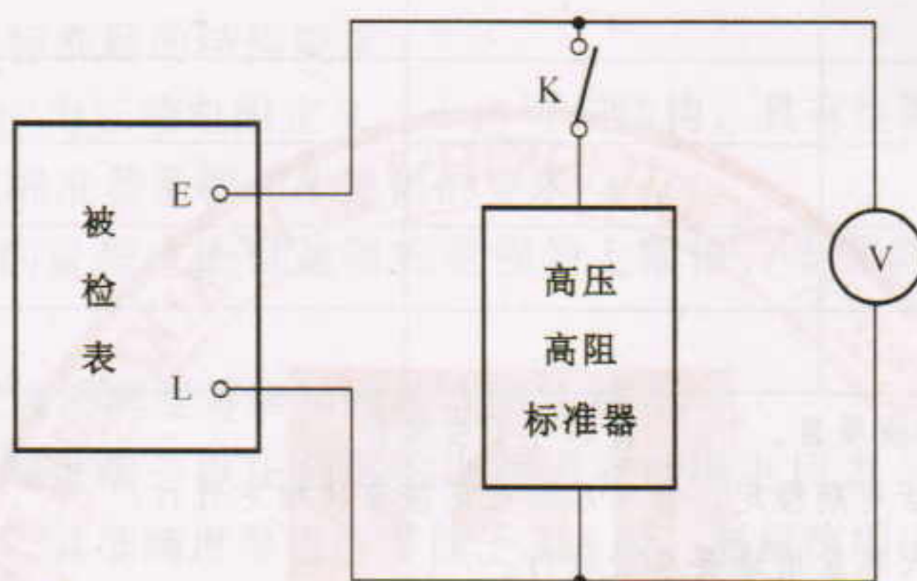
图 2 开路测量电压检定接线图
