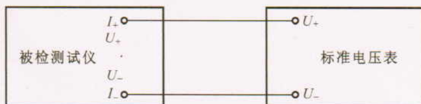
图6 电流源空载电压检定原理图
