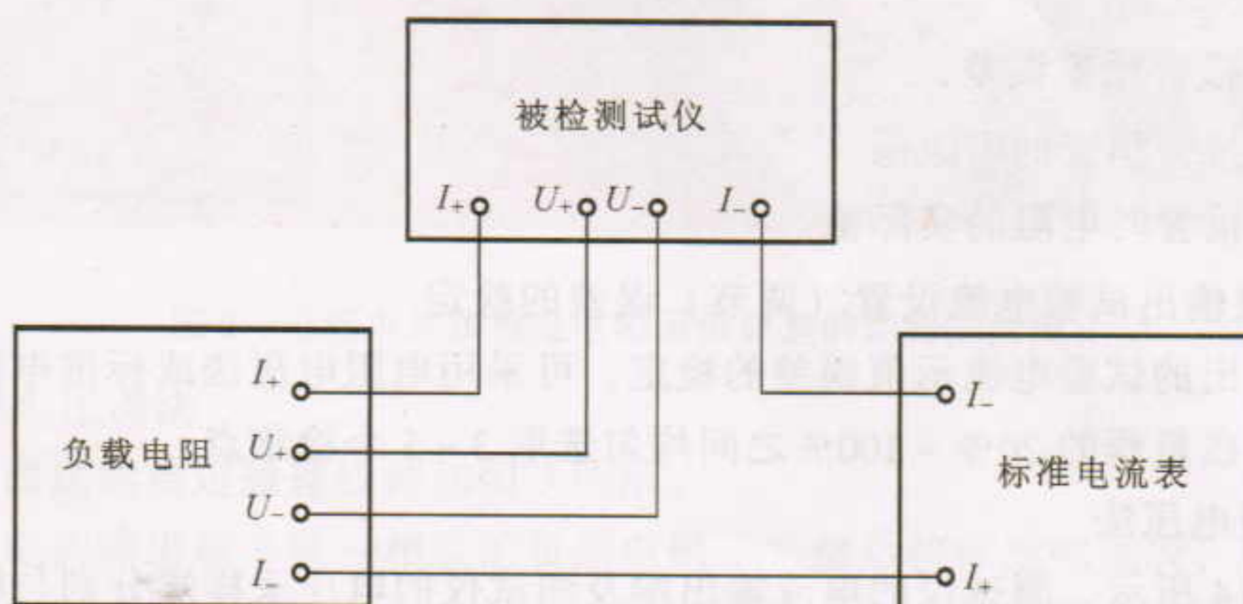
图5 标准电流表法检定测试仪试验电流设置（调节）误差的原理图
