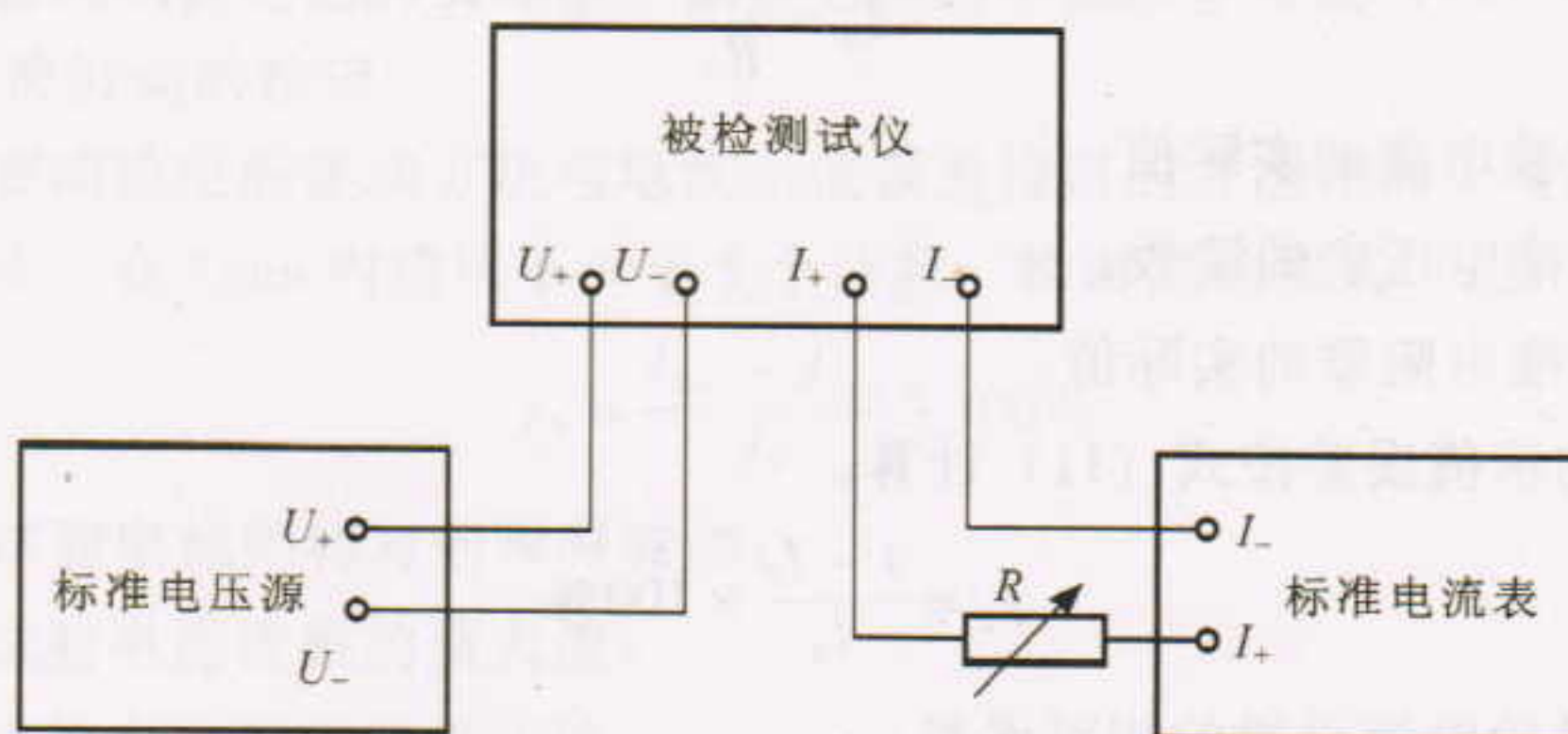
图3 标准电压源法检定电阻示值误差的原理线路图
