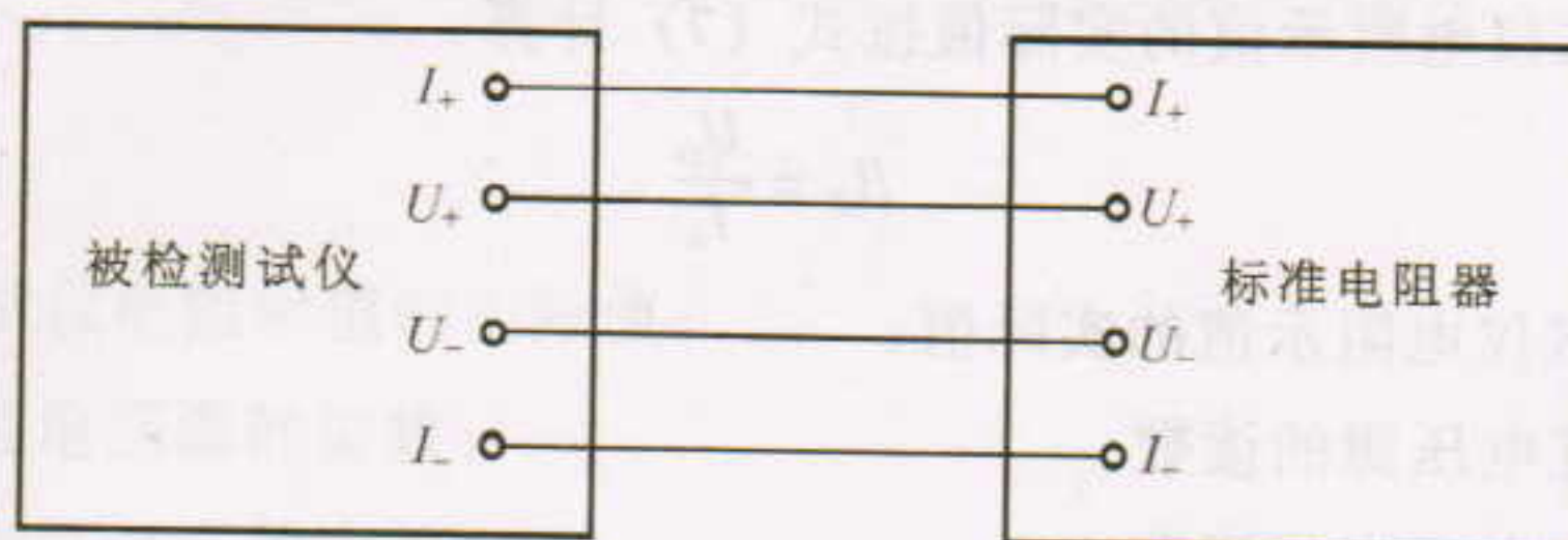
图1 标准电阻器法检定电阻示值误差的原理线路
