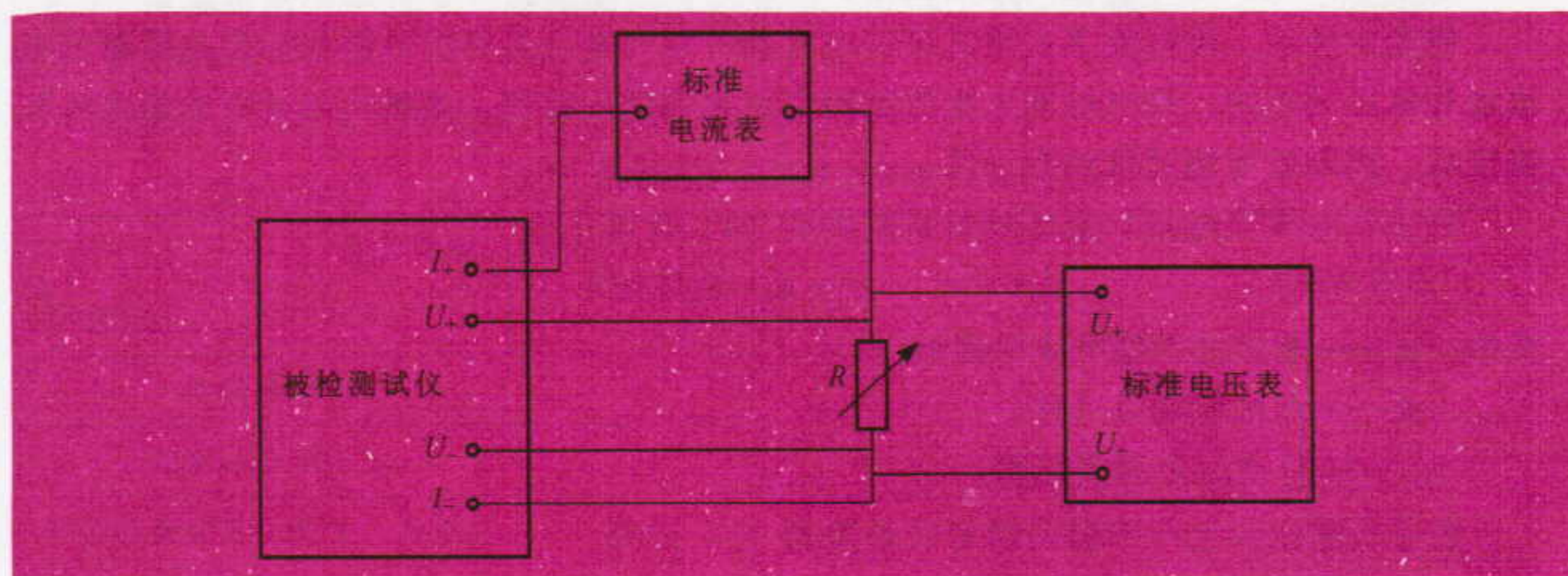
图 2 电流电压法检定电阻示值误差的原理线路图
