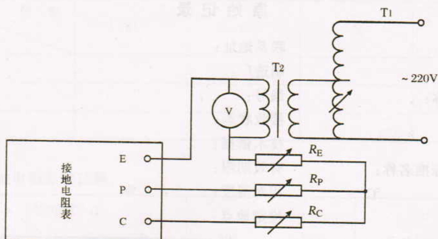
图3 地电压影响试验原理图
