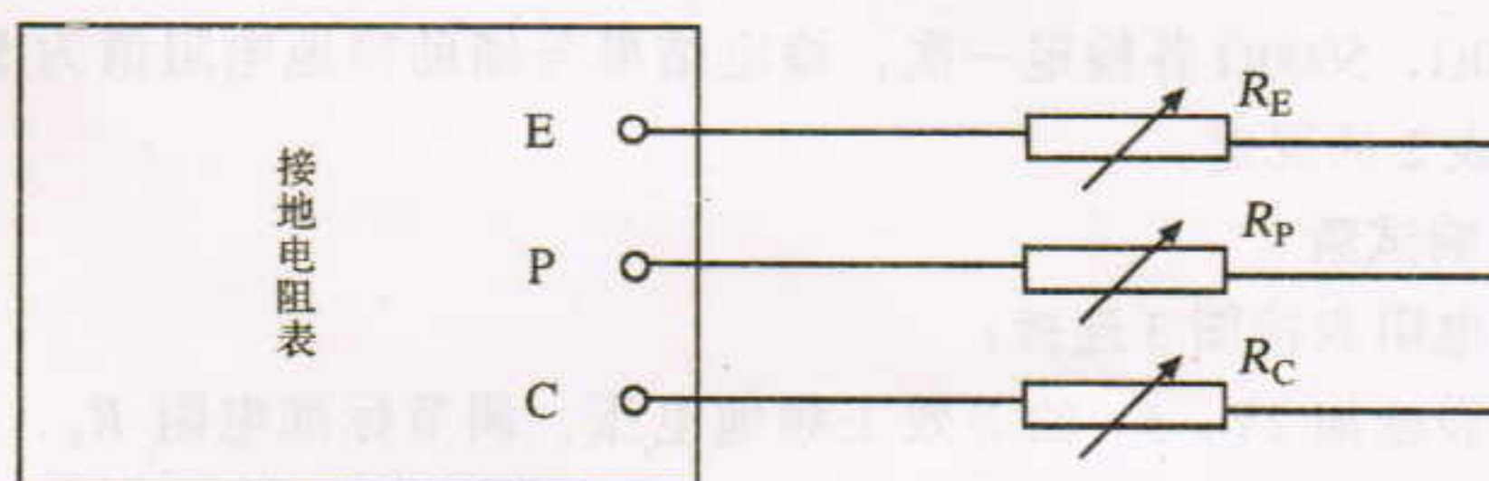
图 1 R_x > 10\Omega 时的原理接线图
