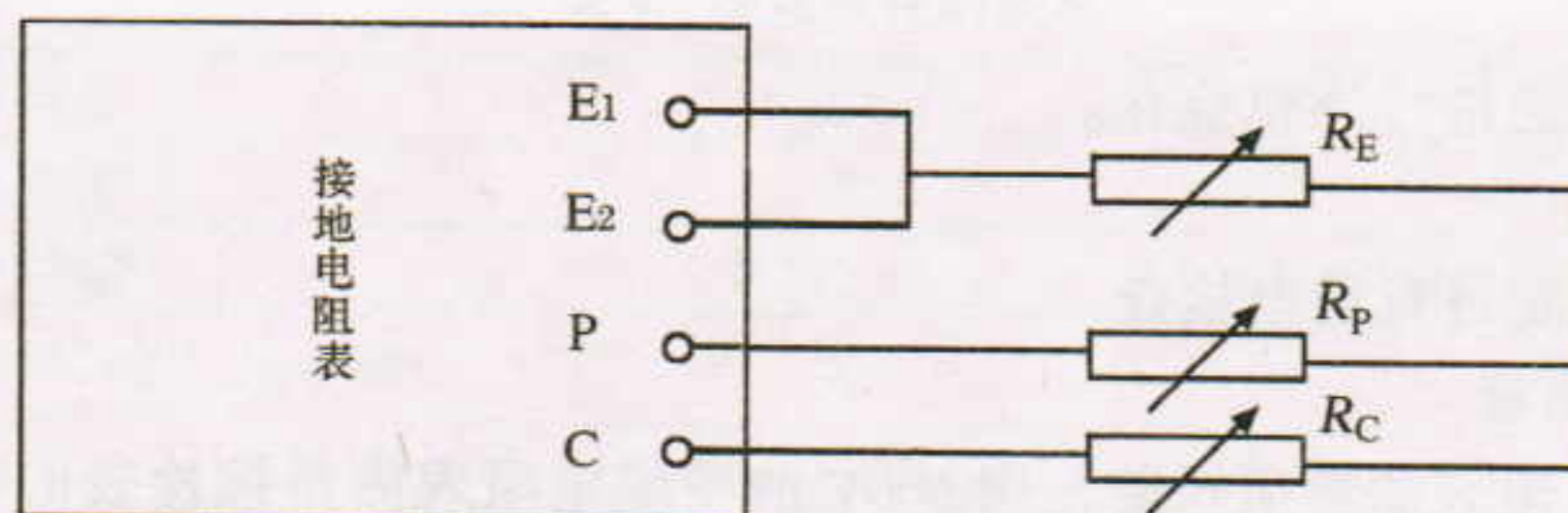
图2 R_x \leq 10\Omega 时的原理接线图
