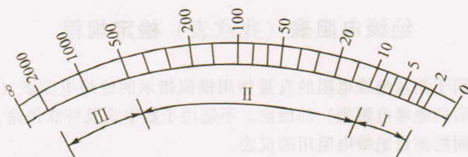
图1 绝缘电阻表量程区段
