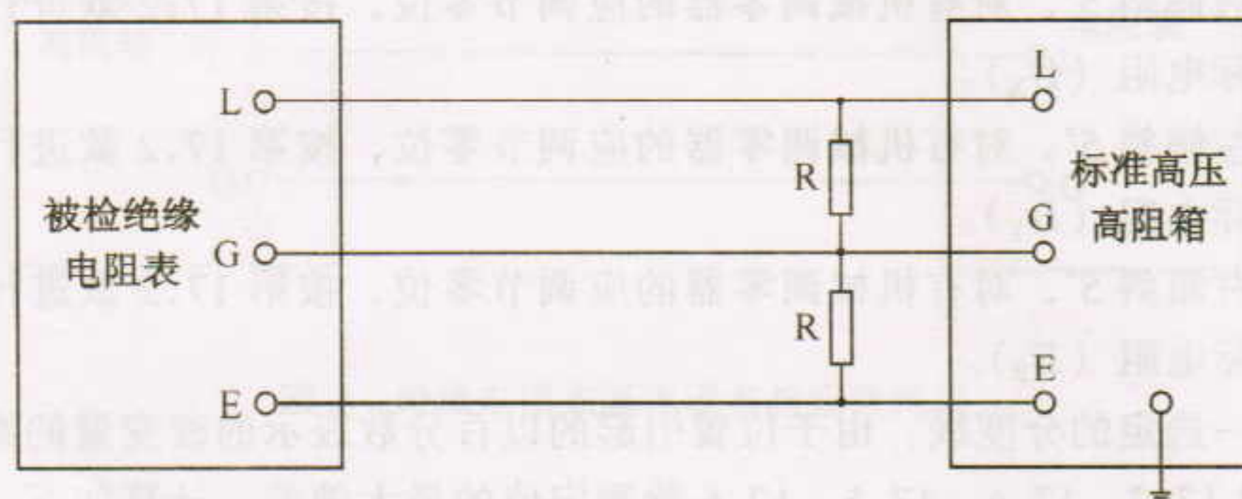
图 4 检查屏蔽装置作用的接线图
