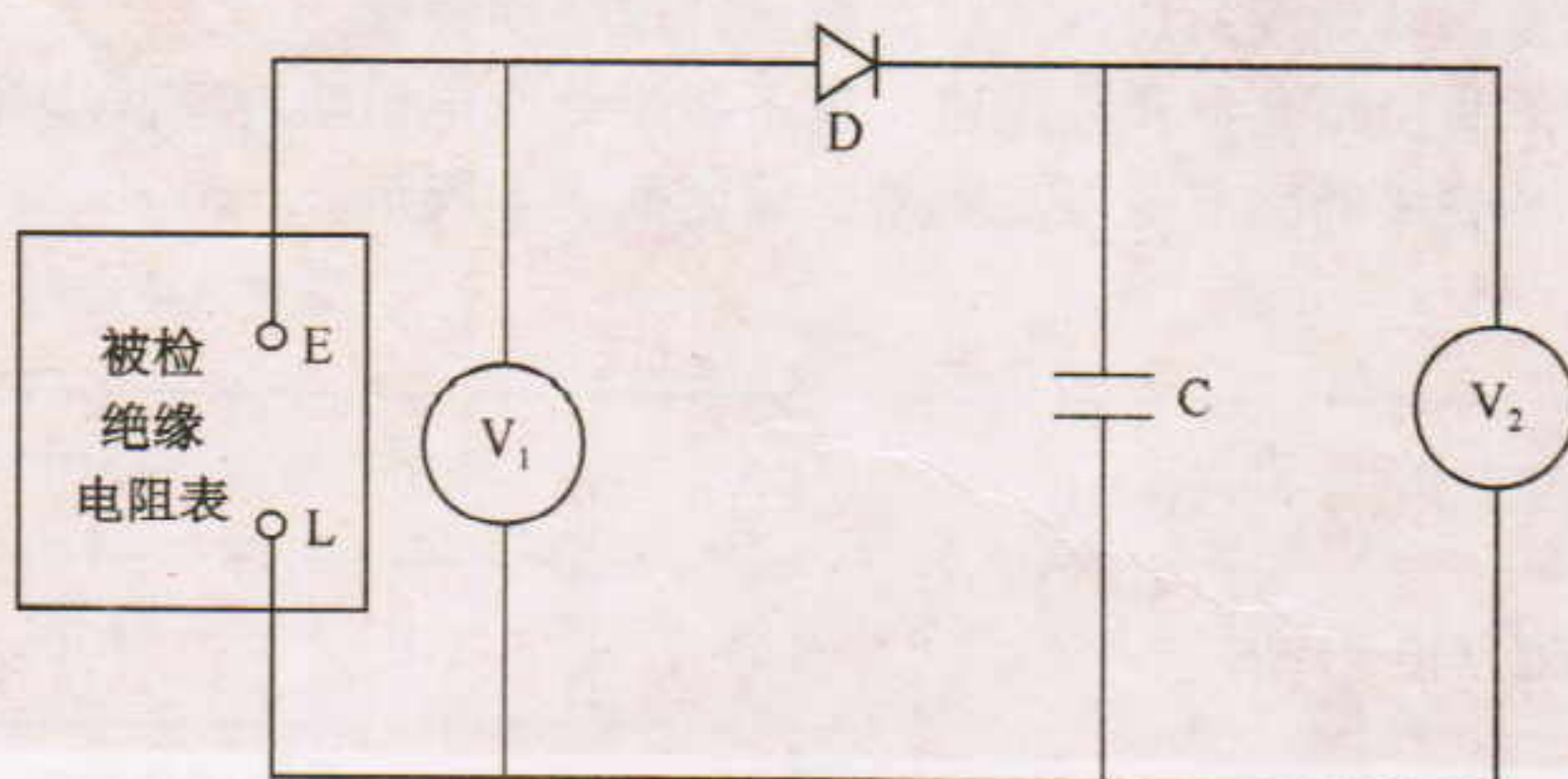
图2 绝缘电阻表基本误差检定接线图
