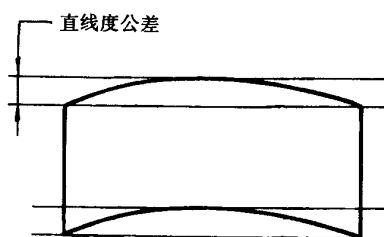
平行度误差 \leq 直线度公差
