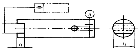
c) 基准:较长要素( l_2 )
