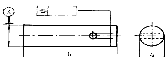
d) 基准:较长要素( l_1 )
