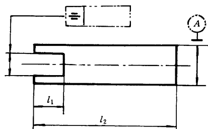
a) 基准:较长要素( l_2 )
