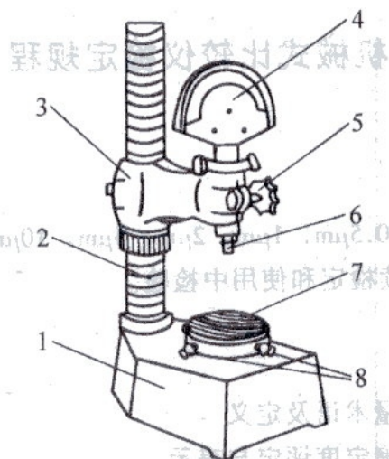
图3 可调式工作台式
