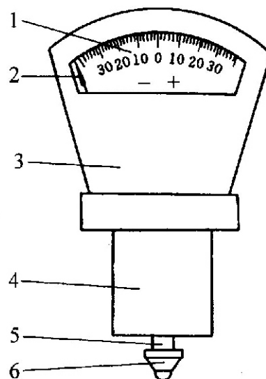
图 2 杠杆式或杠杆齿轮式
