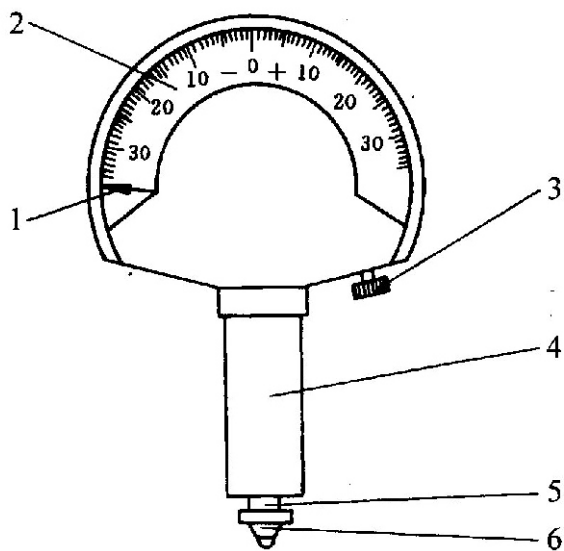
图 1 杠杆齿轮式
