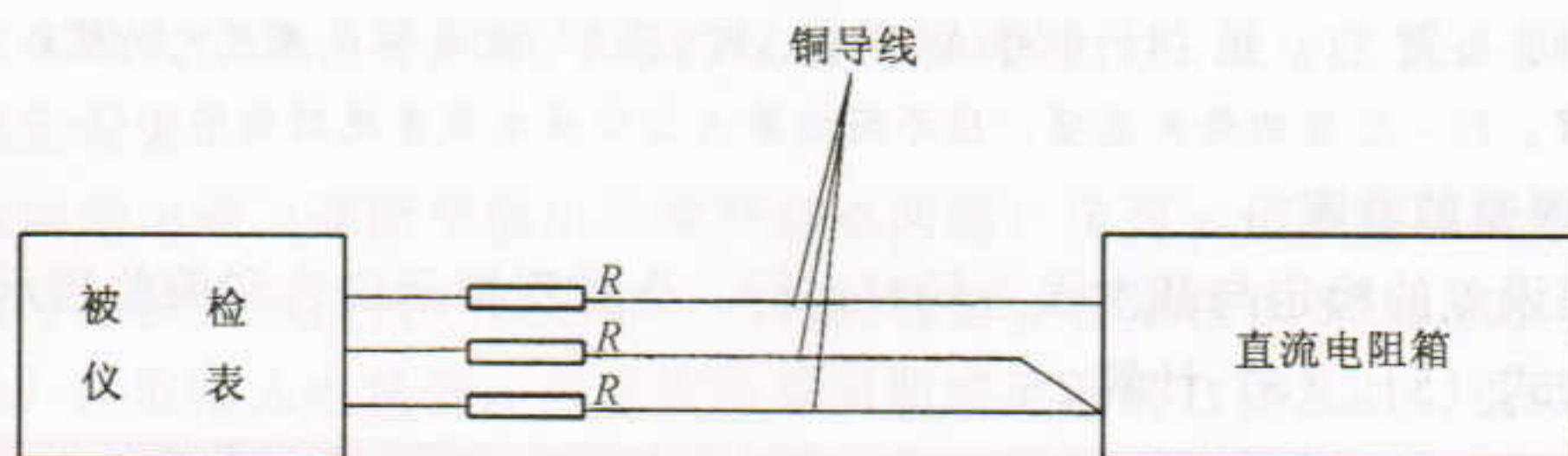
(a) 配三线制热电阻
