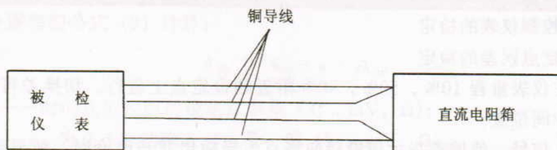
(a) 配三线制热电阻
