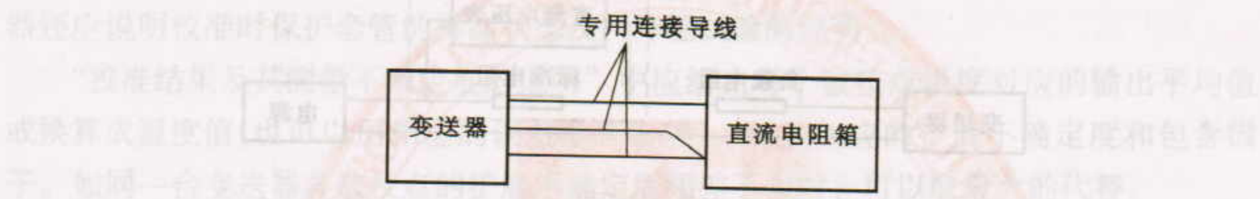
图 A.5 热电阻输入的变送器的测量接线示意图
