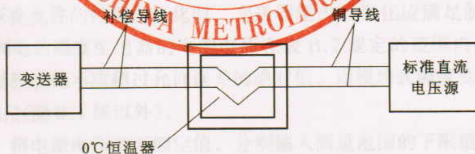
图 A.3 补偿导线法测量接线示意图
