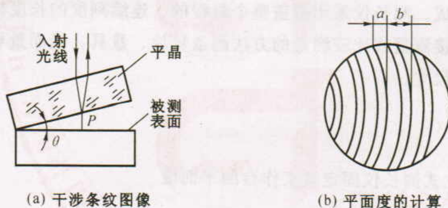
图 1 光波干涉原理示意图
