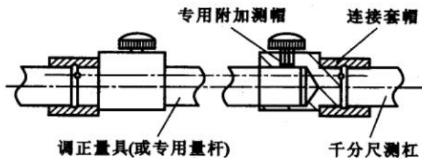
图 10 检平行度的钢球检具
