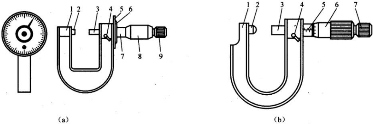
图5 板厚千分尺
