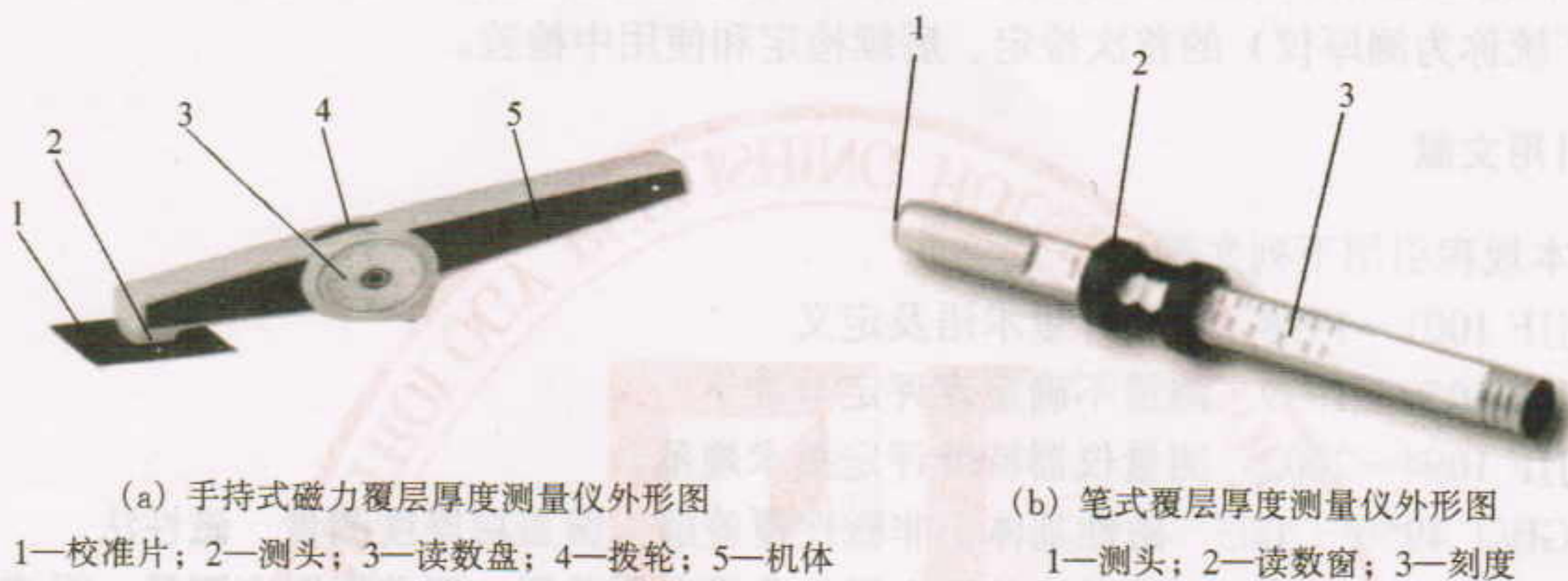
图 2 磁力式覆层厚度测量仪外形图
