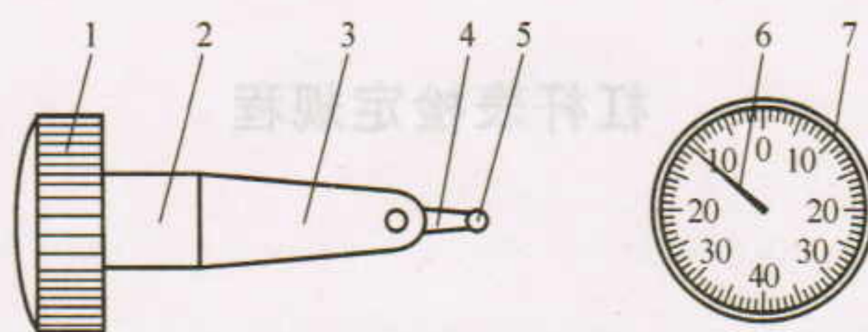
1—表圈；2—夹持柄；3—表体；4—测杆；5—测头；6—指针；7—表盘
