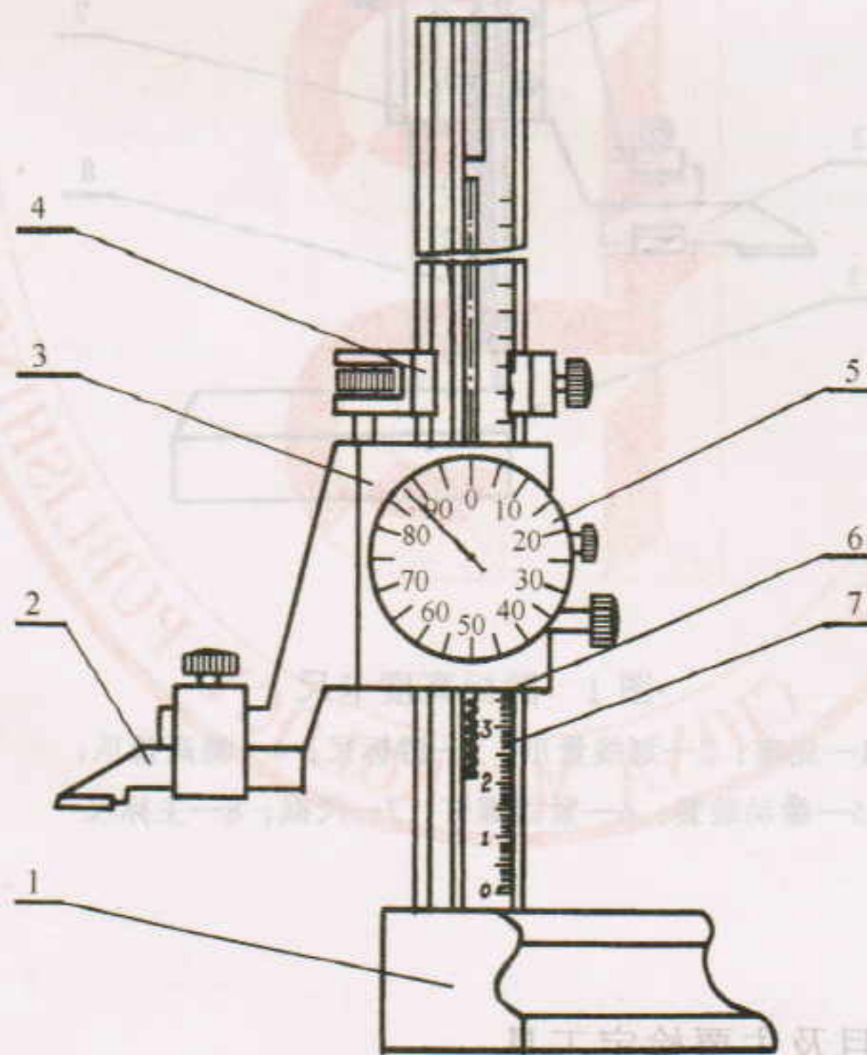
图3 圆标高度卡尺
