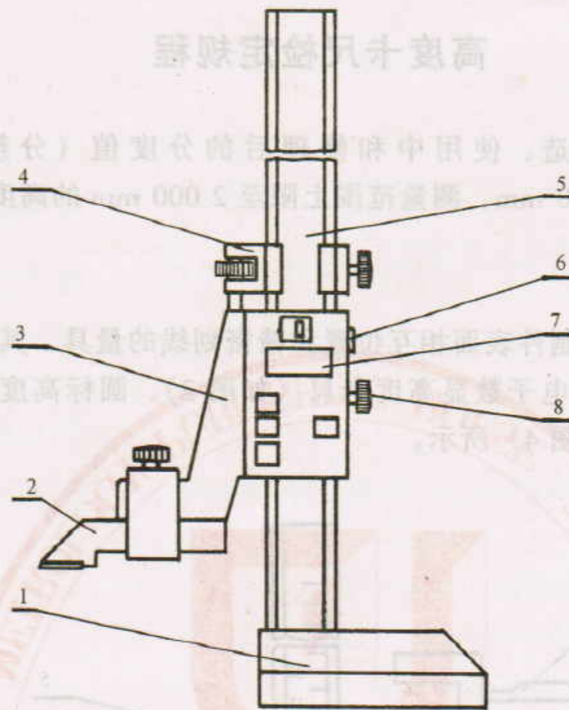
图2 电子数显高度卡尺
