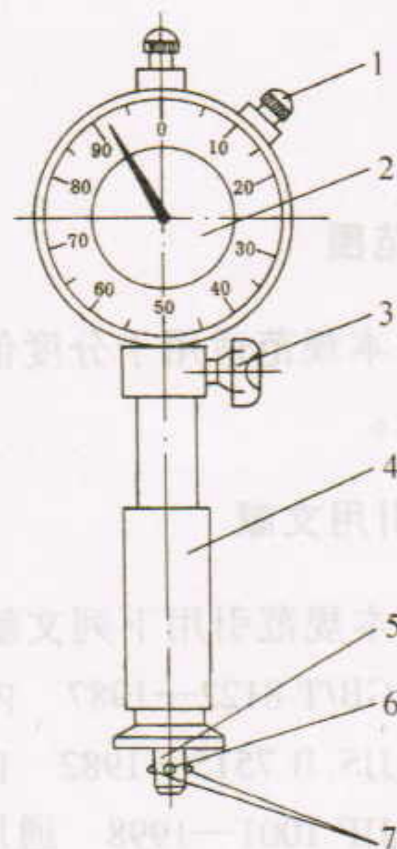
图3 钢球式内径表
