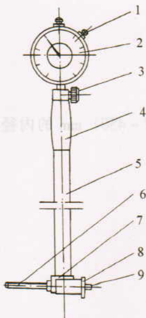
图1 带定位护桥内径表
