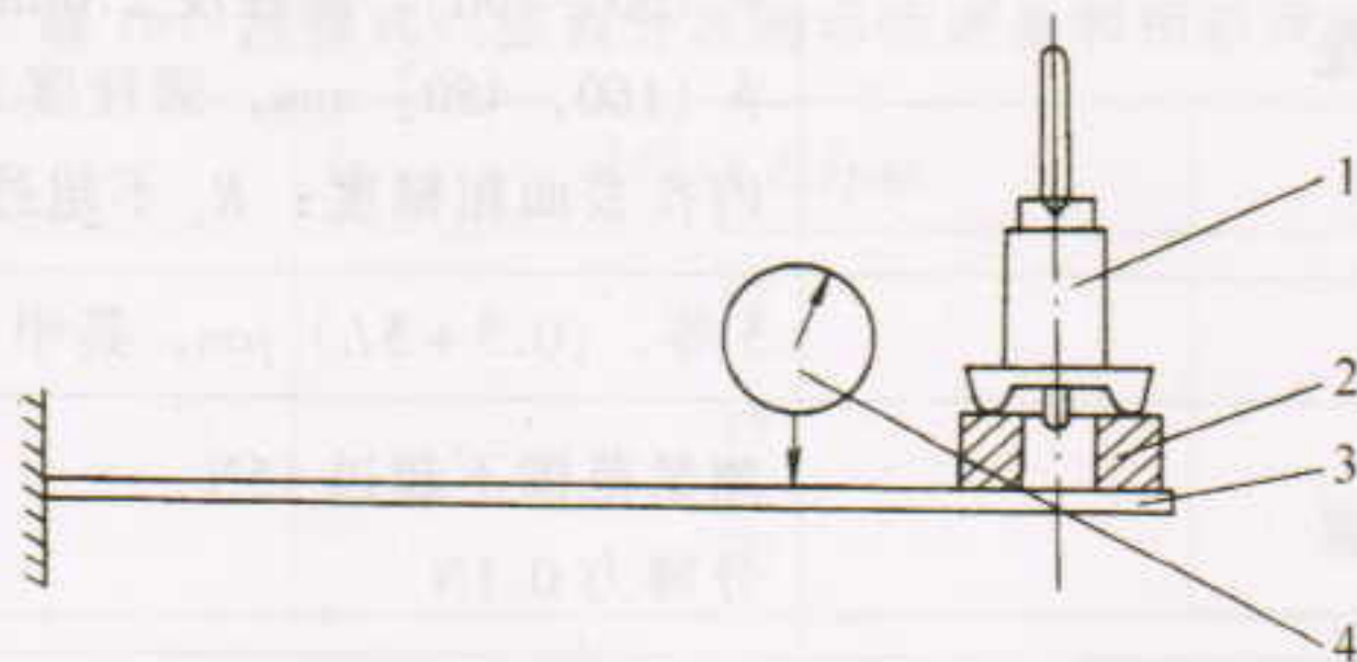
图4 定位护桥接触压力校准示意图
