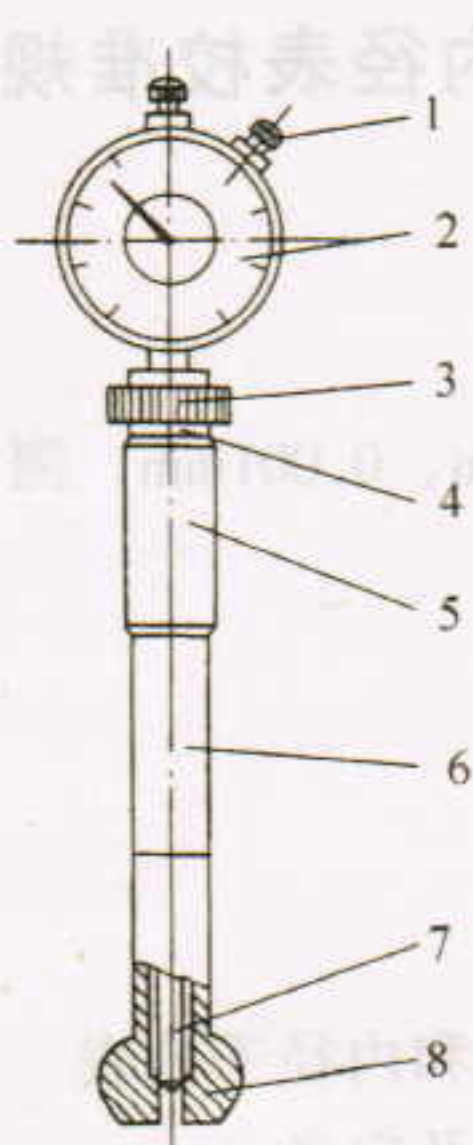
图2 涨簧式内径表
