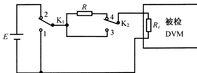
图7 输入电阻和零电流的测试
