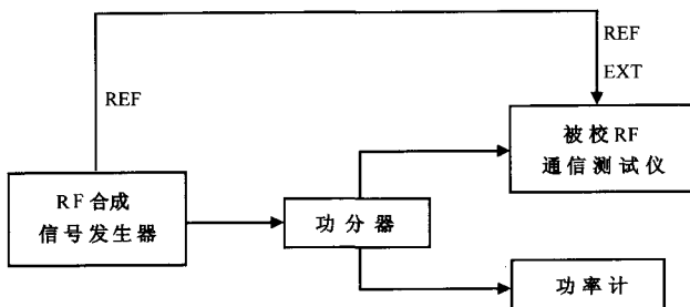
图 4 输入频率响应测试
