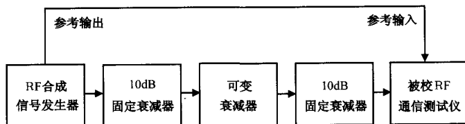
图 3 参考电平范围及准确度校准
