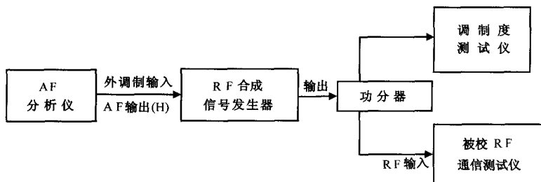
图 13 调制度测量误差的测试
