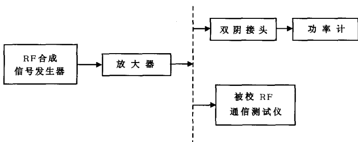
图 12 功率计校准
