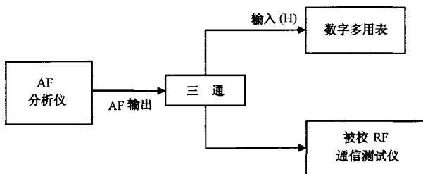
图 18 AC 电压表测量误差的校准
