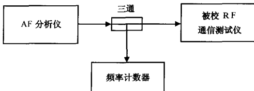
图 17 频率测量误差的校准
