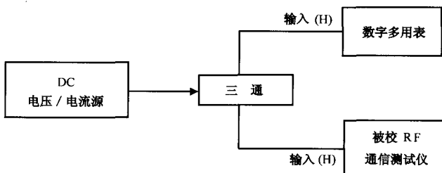
图 19 DC 电压测量误差的校准
