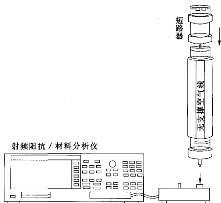
图9 “短路无支撑空气线”阻抗测量示值的校准
