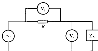
图 1 I - V 测量简化电路
