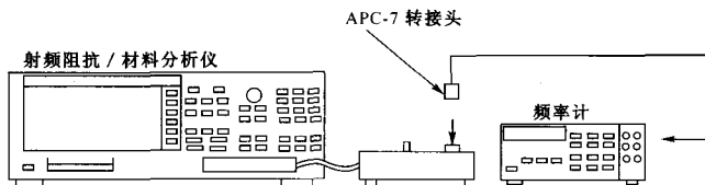
图 2 频率准确度校准连接图
