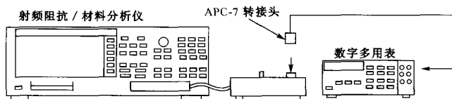
图 4-1 直流偏置电平的校准 (常温)
