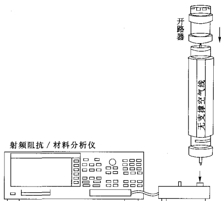
图8 “开路无支撑空气线”阻抗测量示值的校准
