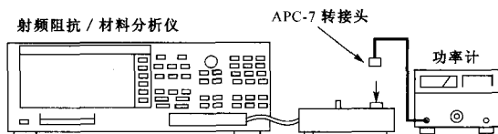
图 3-1 信号电平准确度校准连接图（常温）
