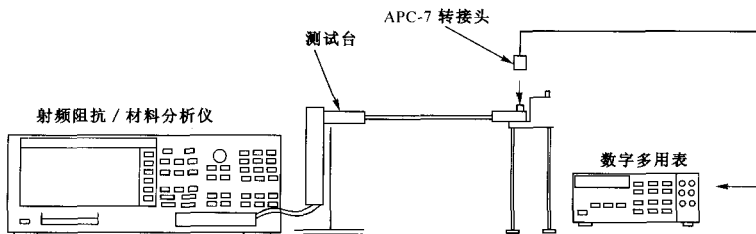
图 4-1 直流偏置电平的校准 (常温)
