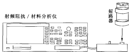
图6 “短路器”阻抗测量值的校准
