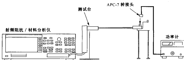
图 3-1 信号电平准确度校准连接图（常温）
