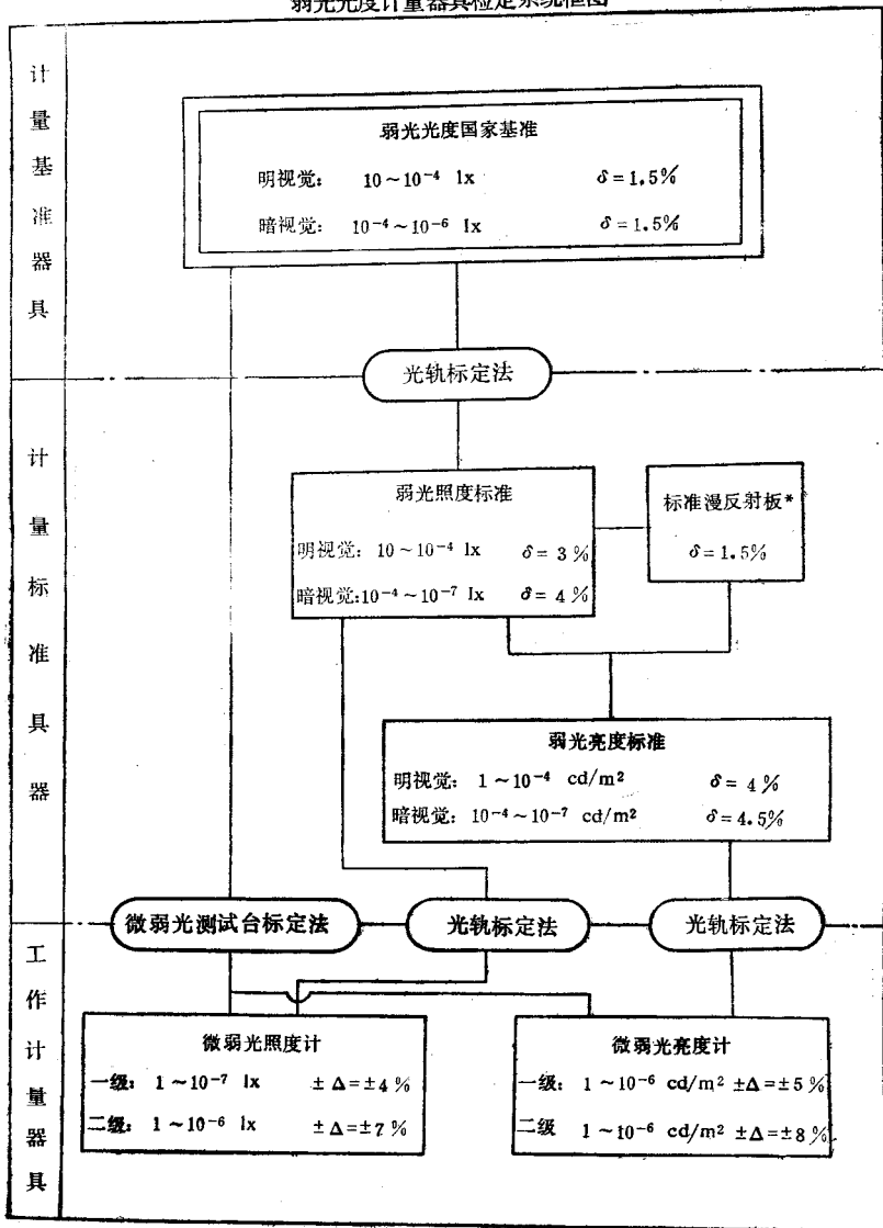
弱光光度计量器具检定系统框图
