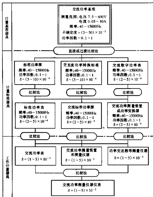
交流功率计量器具检定系统框图
