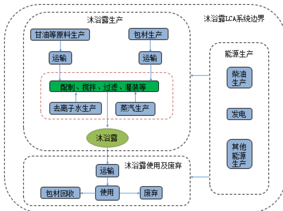
图 B.1 沐浴露产品系统边界图
